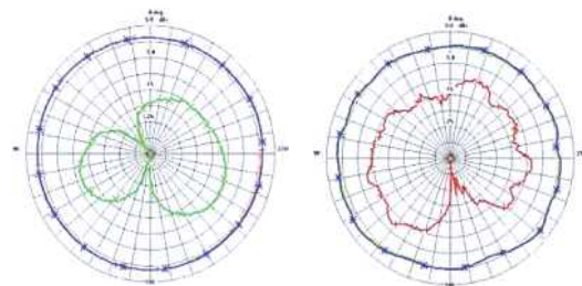
2.4 GHz
