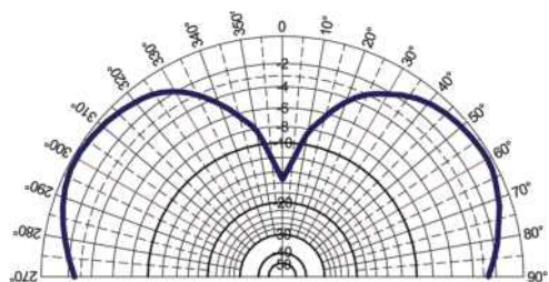
2.4 GHz ■ E-Plane
